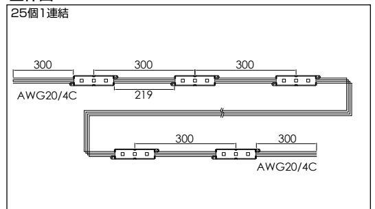
全体図
