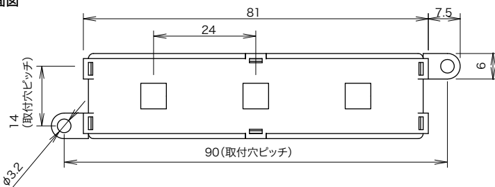
正面図
